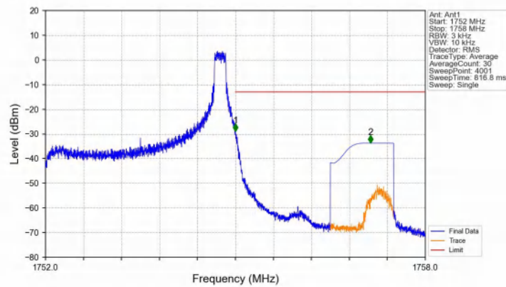
Band4_3MHz_QPSK_HCH_1753.5MHz_RB_1_14_NTNV
