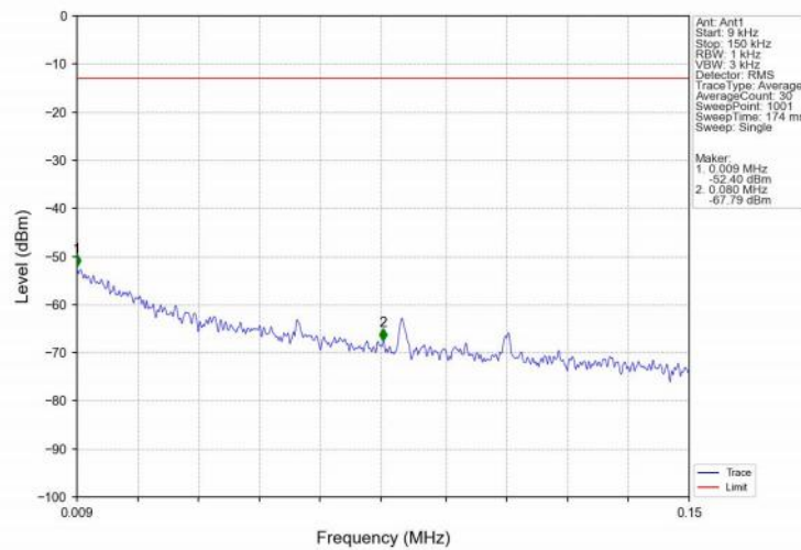
Band4_15MHz_QPSK_LCH_1717.5MHz_RB_1_0_NTNV
