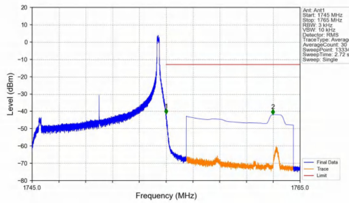
Band4_10MHz_QPSK_HCH_1750MHz_RB_1_49_NTNV
