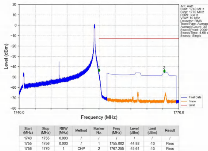
Band4_15MHz_QPSK_HCH_1747.5MHz_RB_1_74_NTNV
