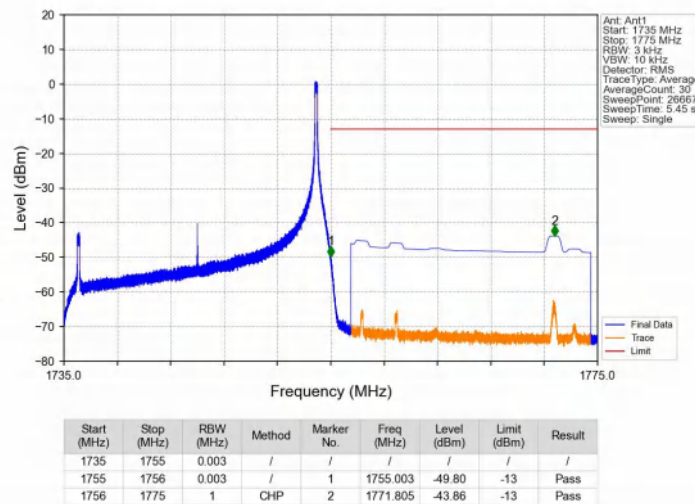
Band4_20MHz_QPSK_HCH_1745MHz_RB_1_99_NTNV
