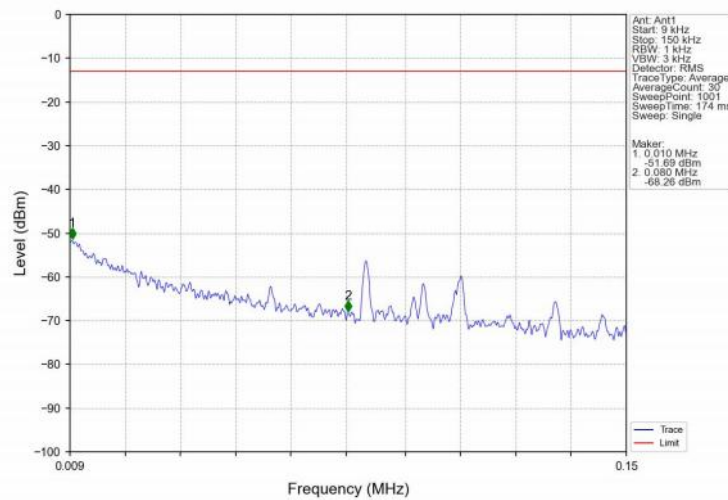
Band4_20MHz_QPSK_LCH_1720MHz_RB_1_0_NTNV
