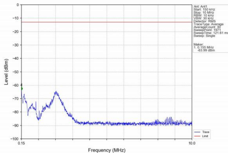
Band2_10MHz_16QAM_MCH_1880MHz_RB_1_0_NTNV
