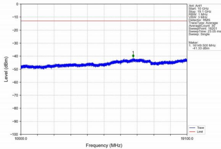
Band2_15MHz_QPSK_HCH_1902.5MHz_RB_1_74_NTNV
