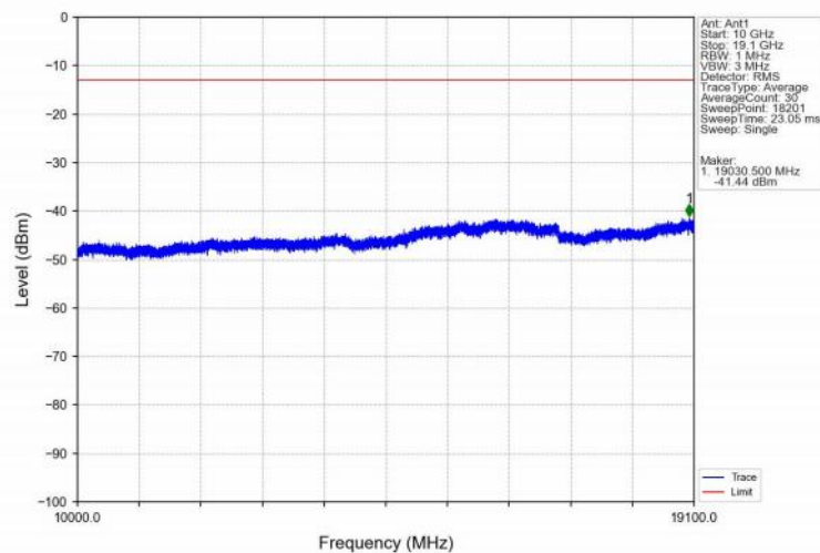
Band2_10MHz_QPSK_MCH_1880MHz_RB_1_0_NTNV
