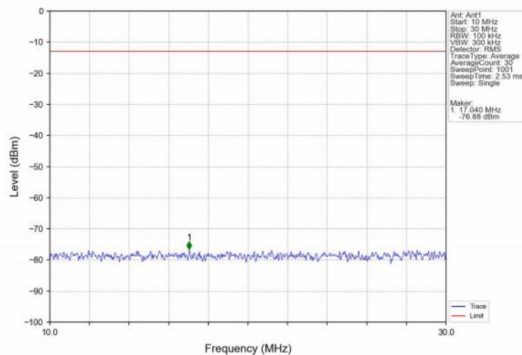
Band2_10MHz_QPSK_MCH_1880MHz_RB_1_0_NTNV
