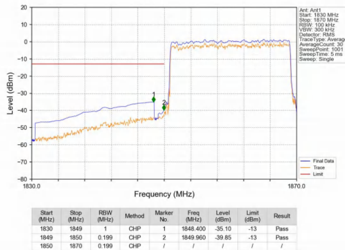
Band2_20MHz_16QAM_LCH_1860MHz_RB_100_0_NTNV
