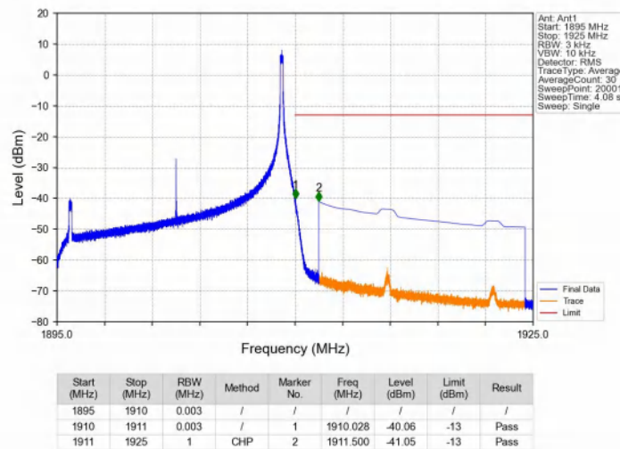
Band2_15MHz_QPSK_HCH_1902.5MHz_RB_1_74_NTNV
