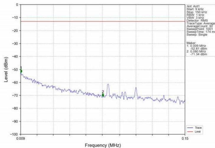
Band2_20MHz_16QAM_HCH_1900MHz_RB_1_0_NTNV
