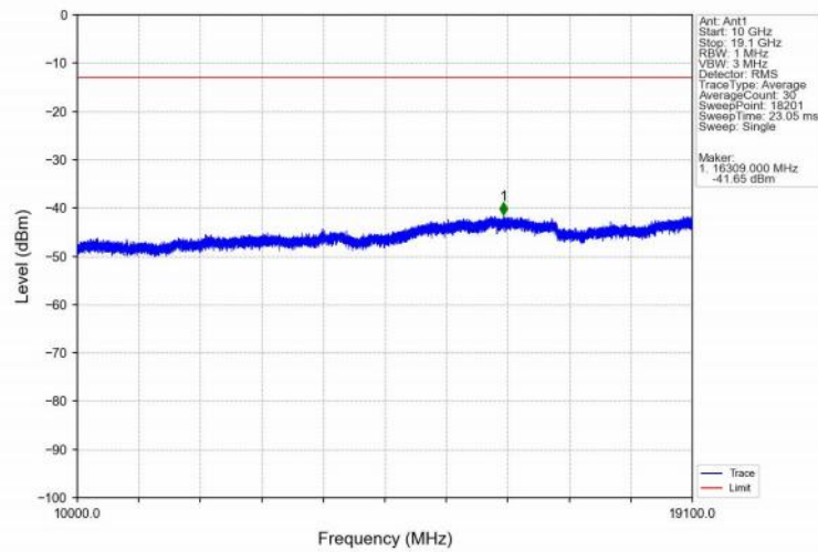
Band2_3MHz_QPSK_HCH_1908.5MHz_RB_1_14_NTNV
