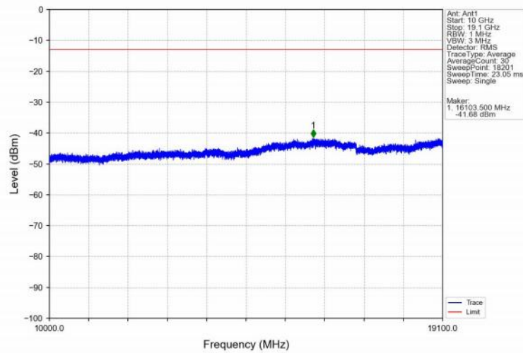
Band2_20MHz_QPSK_HCH_1900MHz_RB_1_99_NTNV
