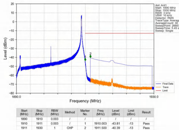
Band2_20MHz_QPSK_HCH_1900MHz_RB_1_99_NTNV
