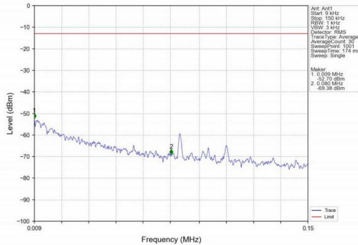
Band2_20MHz_QPSK_LCH_1860MHz_RB_1_0_NTNV
