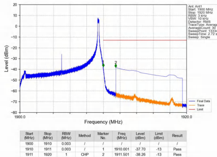
Band2_10MHz_QPSK_HCH_1905MHz_RB_1_49_NTNV
