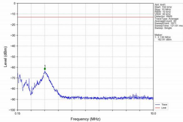
Band2_20MHz_QPSK_LCH_1860MHz_RB_1_0_NTNV
