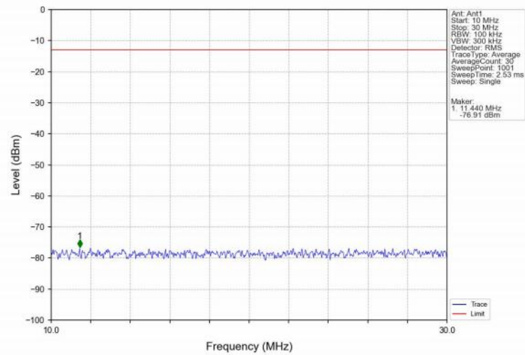
Band2_20MHz_QPSK_HCH_1900MHz_RB_1_0_NTNV
