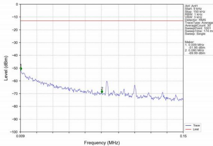
Band2_15MHz_QPSK_LCH_1857.5MHz_RB_1_0_NTNV
