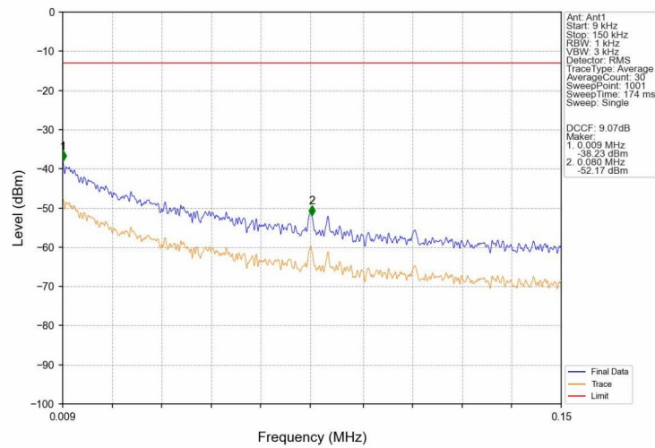
GSM850_GSM_HCH_848.8MHz_GSM_NTNV
