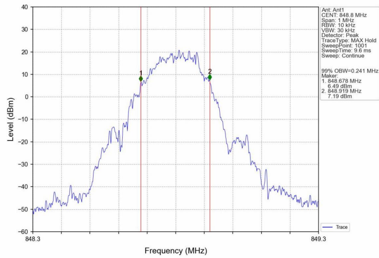
GSM850_EGPRS_HCH_848.8MHz_1 TX Slot_NTNV
