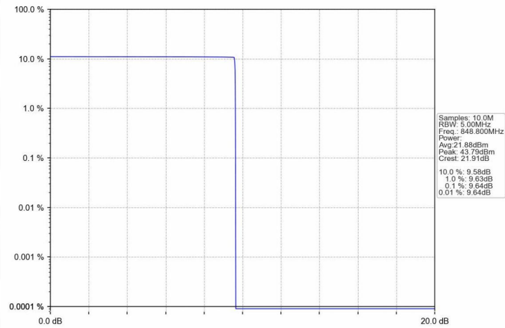
GSM850_GSM_HCH_848.8MHz_GSM_NTNV
