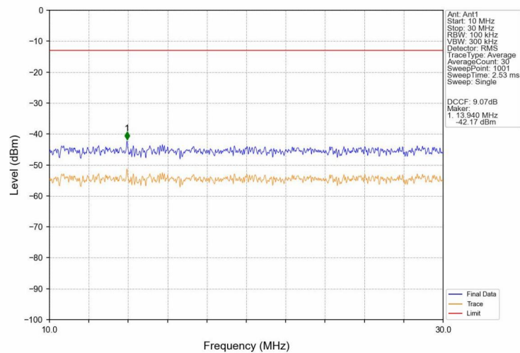
GSM850_GSM_LCH_824.2MHz_GSM_NTNV
