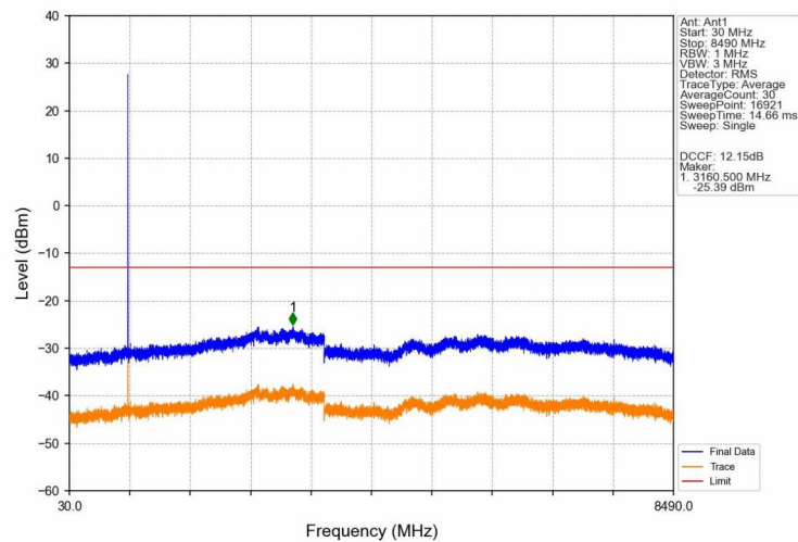
GSM850_EGPRS_HCH_848.8MHz_1 TX Slot_NTNV
