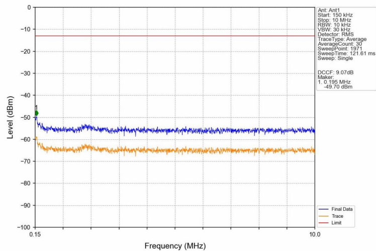
GSM850_GSM_HCH_848.8MHz_GSM_NTNV
