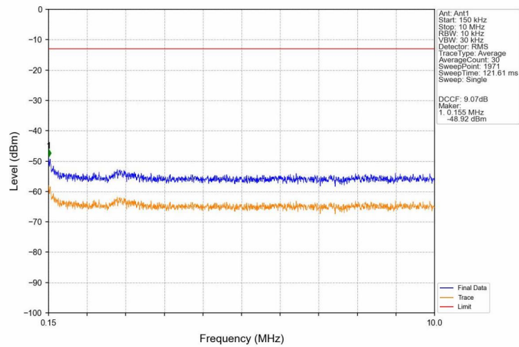
GSM850_GSM_LCH_824.2MHz_GSM_NTNV
