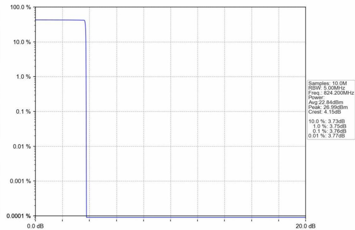
GSM850_GPRS_LCH_824.2MHz_4 TX Slots_NTNV
