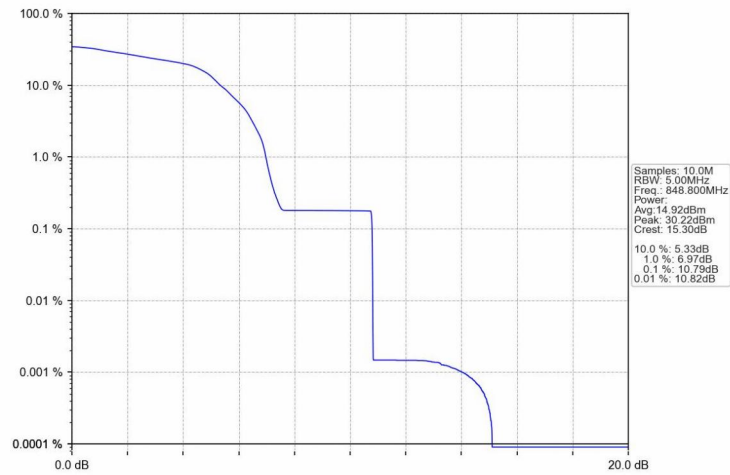
GSM850_EGPRS_HCH_848.8MHz_4 TX Slots_NTNV
