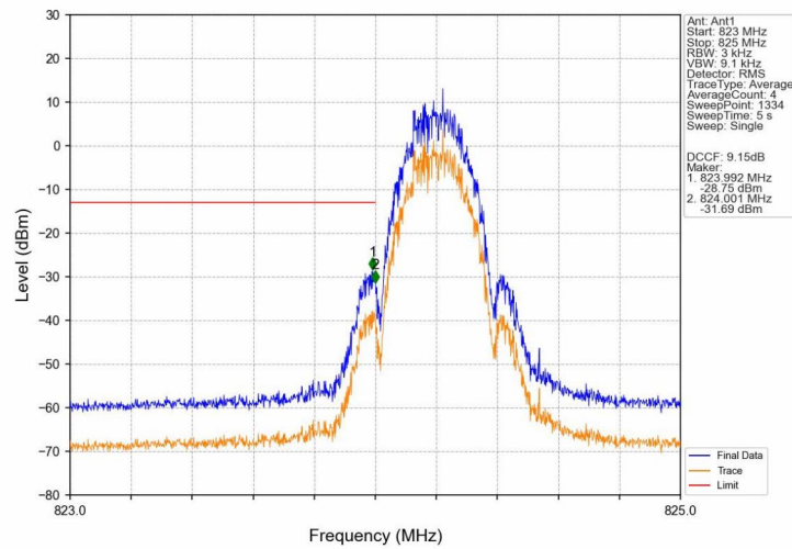
GSM850_EGPRS_LCH_824.2MHz_1 TX Slot_NTNV
