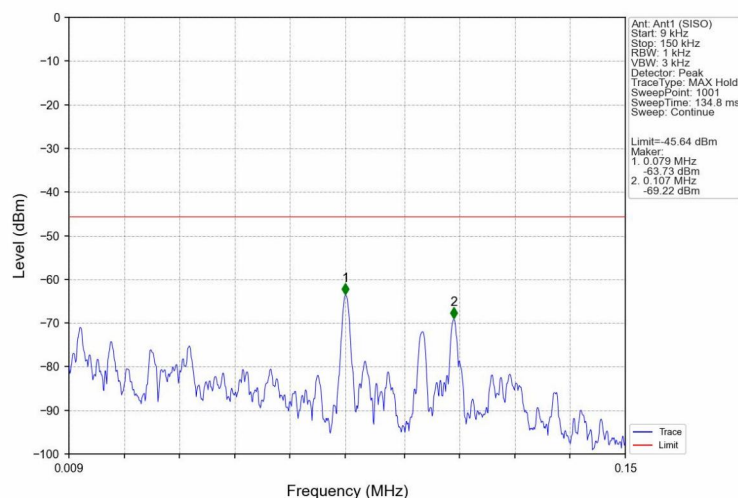
802.11b_HCH_2462MHz_Ant1 (SISO)_NTNV
