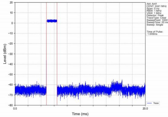
8DPSK_3DH3_HOPP_Ant1_NTNV
