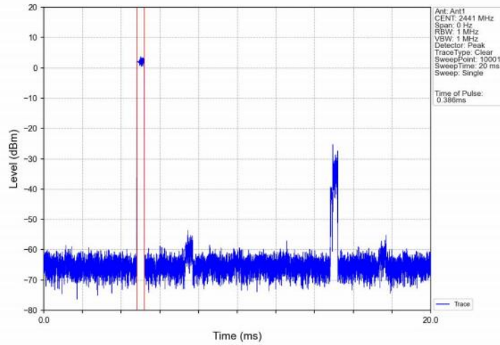
8DPSK_3DH1_HOPP_Ant1_NTNV
