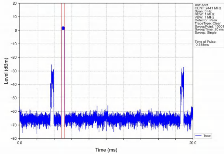
Pi/4DQPSK_2DH1_HOPP_Ant1_NTNV
