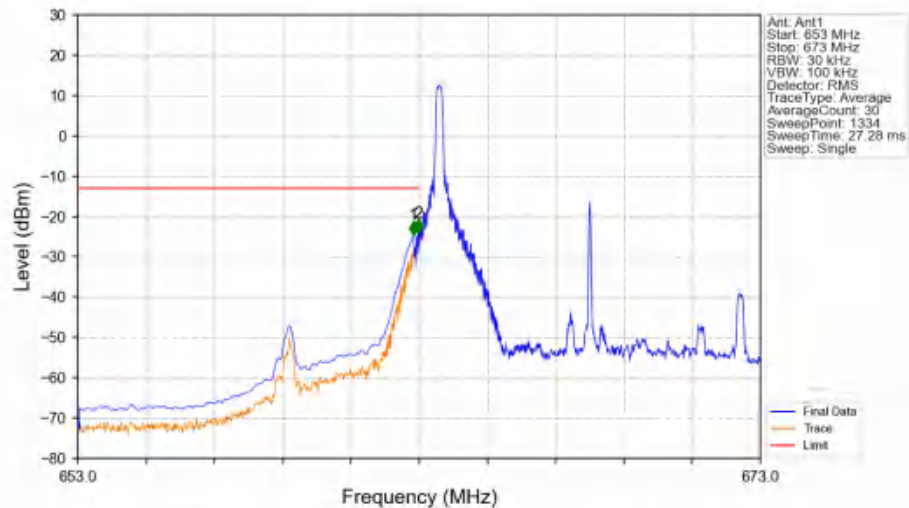
Band71_10MHz_QPSK_LCH_668MHz_RB_1_0_NTNV
