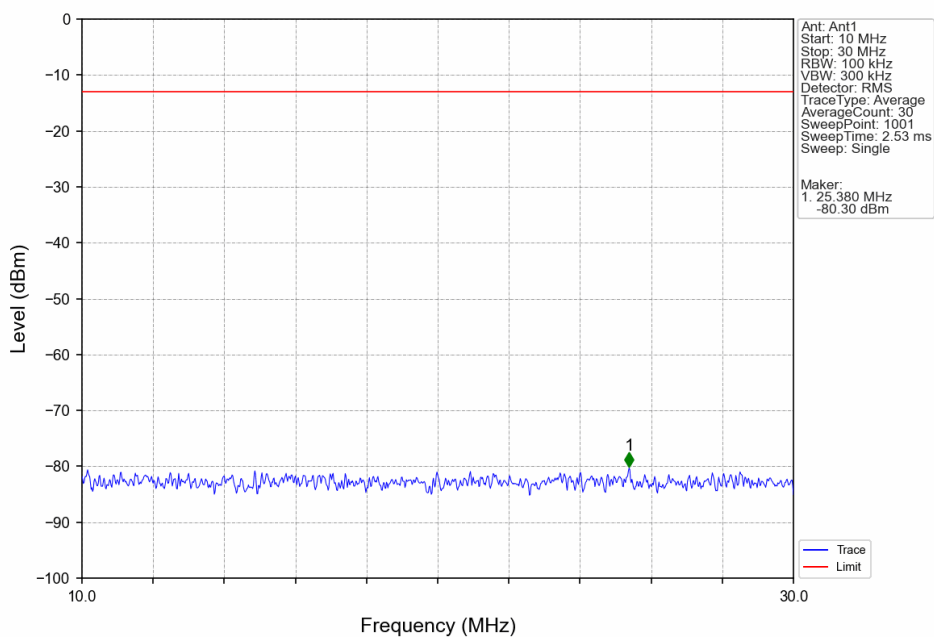
Band17 5MHz QPSK LCH 706.5MHz RB 1 0 NTN
