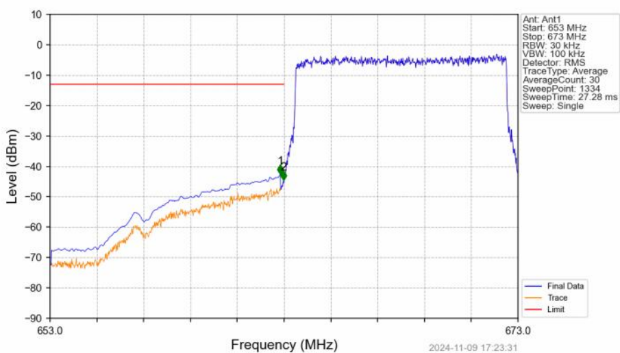
Band71_10MHz_16QAM_LCH_668MHz_RB_50_0_NTNV
