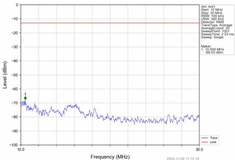
Band66_20MHz_QPSK_MCH_1745MHz_RB_1_0_NTNV
