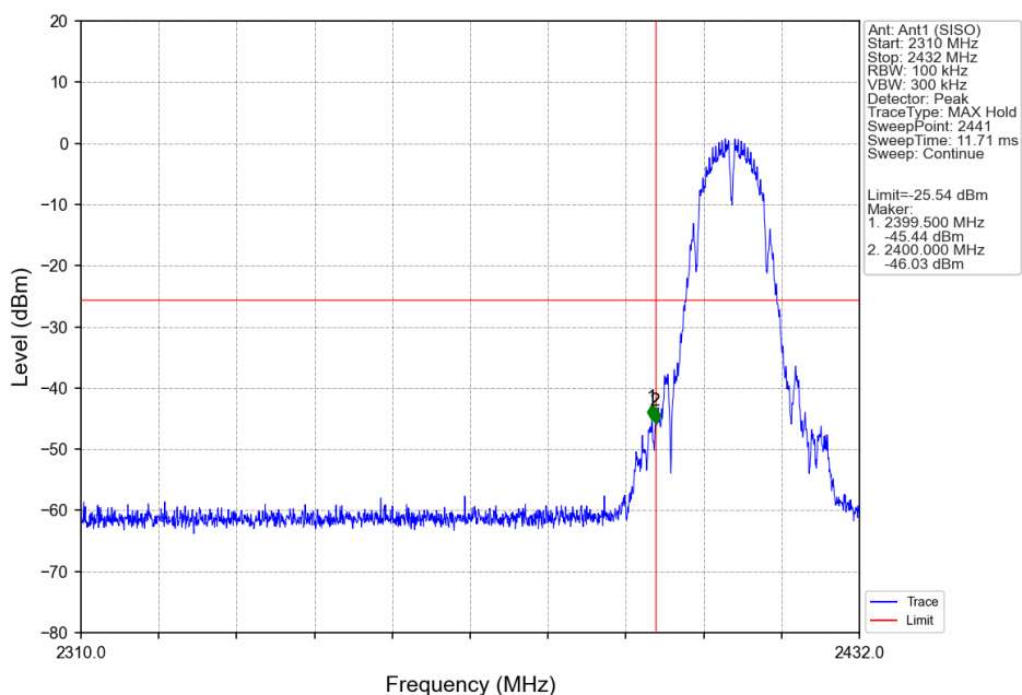
802.11b LCH 2412MHz Ant1 (SISO) NTV
