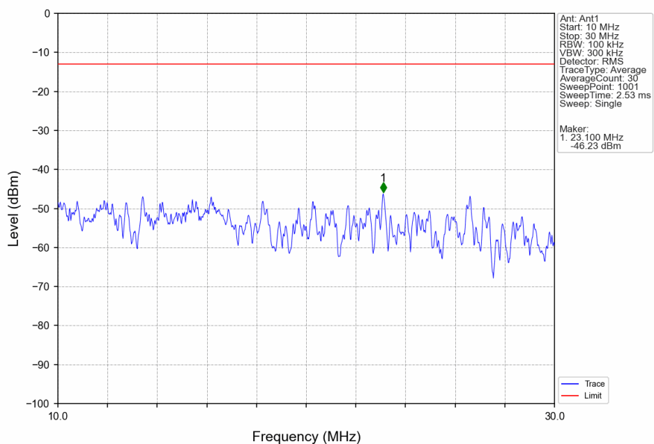
Band71_20MHz_16QAM_LCH_673MHz_RB_1_0 NTN
