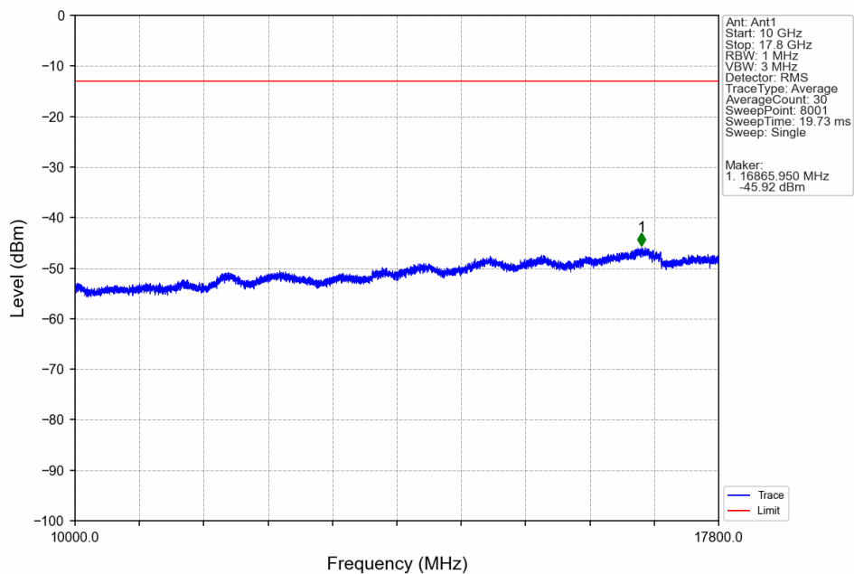
Band66 10MHz QPSK HCH 1775MHz RB 1 49 NTN
