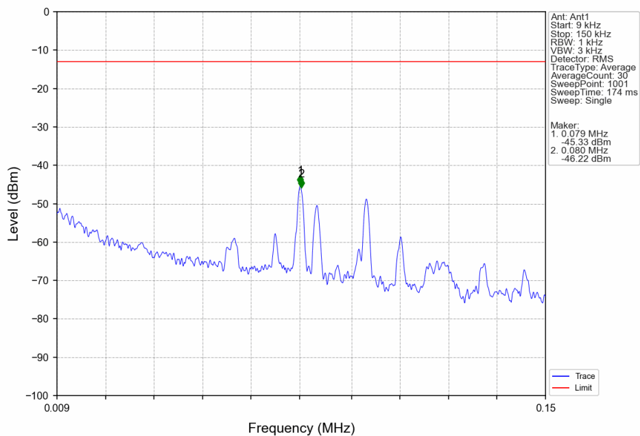
Band66 5MHz 16QAM LCH 1712.5MHz RB 1 0 NTV
