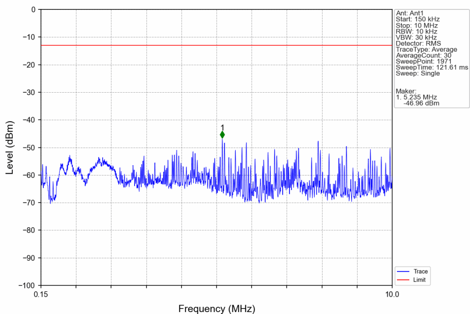
Band66 5MHz 16QAM LCH 1712.5MHz RB 1 0 NTV
