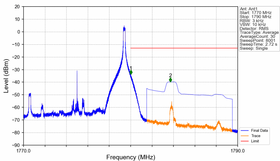
Band66 10MHz QPSK HCH 1775MHz RB 1 49 NTN
