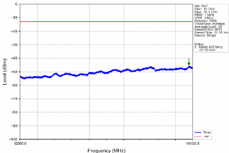
Band2_20MHz_16QAM_LCH_1860MHz_RB_100_0_NTNV
