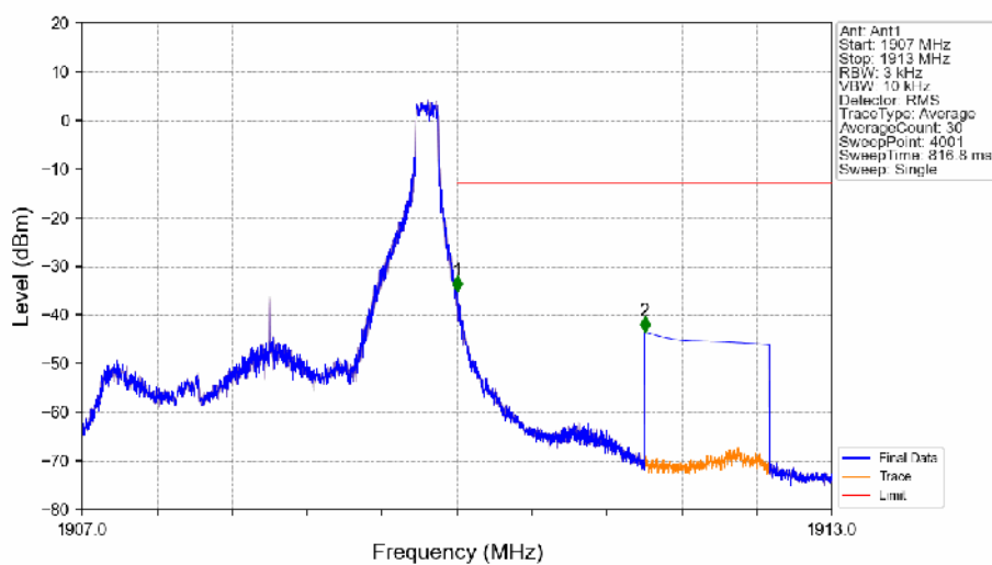
Band2_3MHz_QPSK_HCH_1908.5MHz_RB_1_14_NTNV
