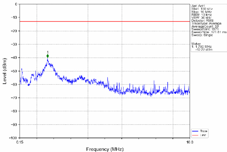
Band2_3MHz_QPSK_MCH_1880MHz_RB_1_0 NTN
