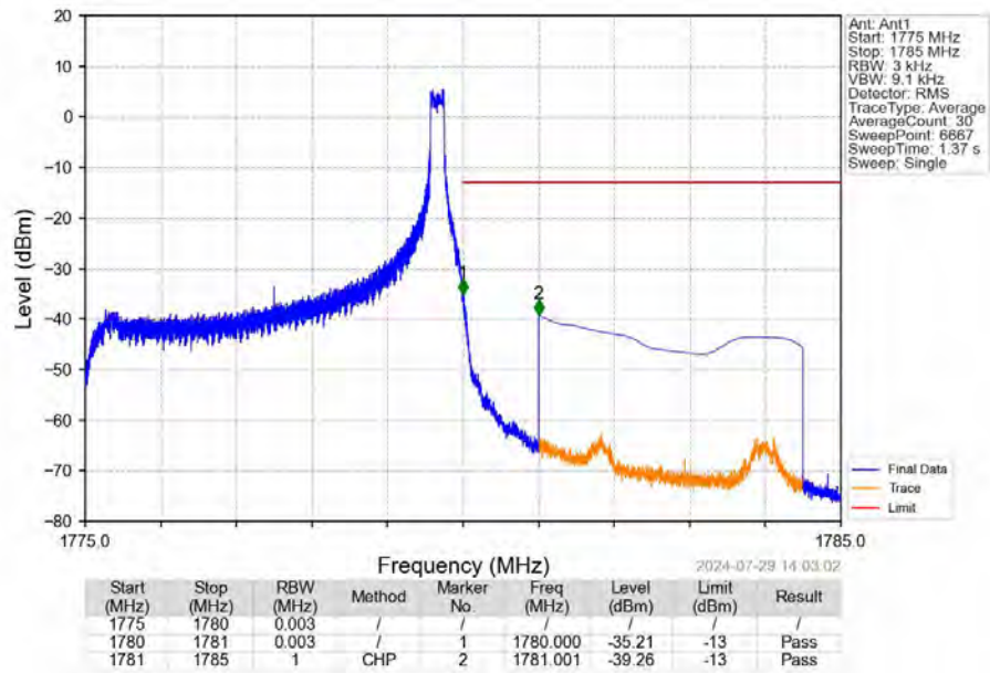
Band66_5MHz_QPSK_HCH_1777.5MHz_RB_1_24_NTNV
