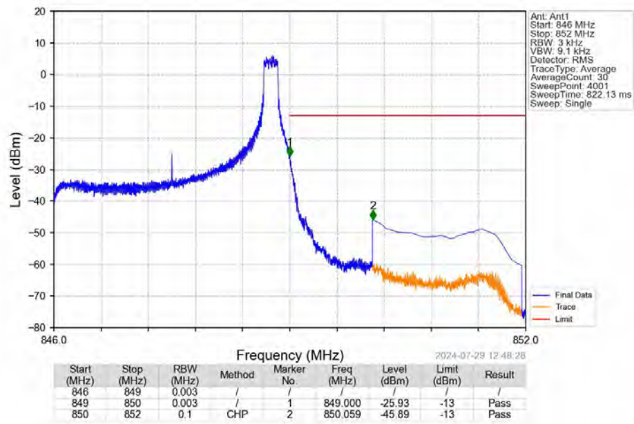
Band26b_3MHz_QPSK_HCH_847.5MHz_RB_1_14_NTNV
