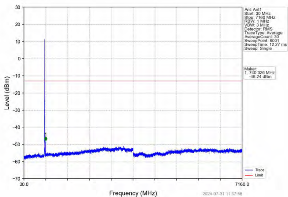
Band17_10MHz_QPSK_MCH_710MHz_RB_1_0_NTNV
