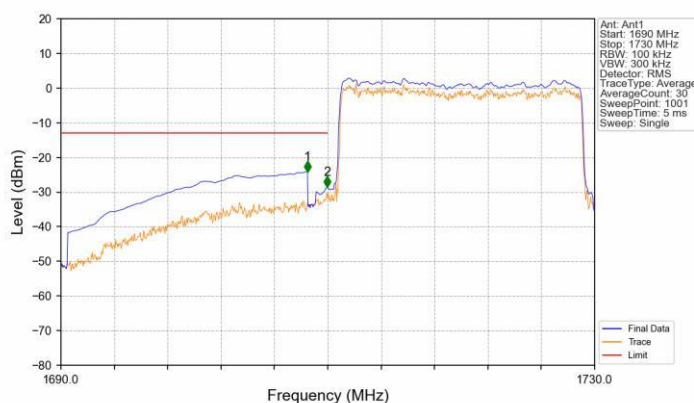
Band66 20MHz 16QAM LCH 1720MHz RB 100 0 NTNV
