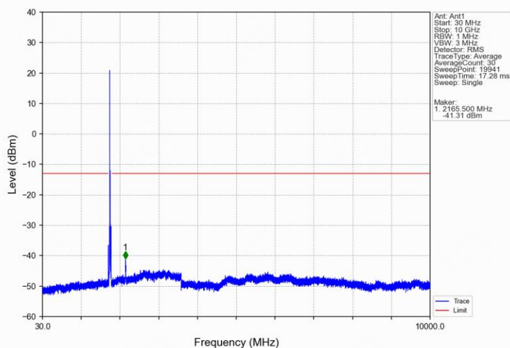
Band66 20MHz 16QAM HCH 1770MHz RB 1 0 NTV
