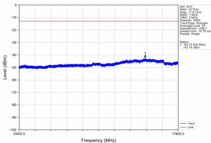
Band66 20MHz 16QAM HCH 1770MHz RB 1 0 NTV
