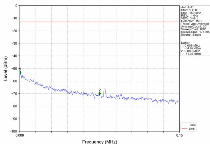
Band66 20MHz 16QAM HCH 1770MHz RB 1 0 NTNV
