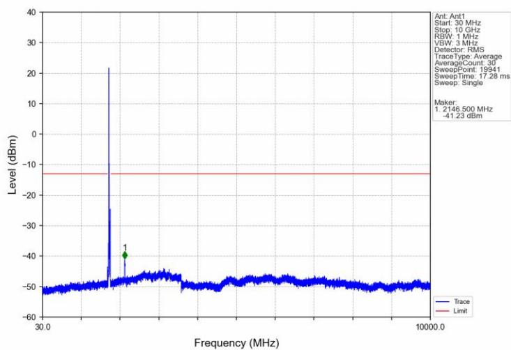
Band66 20MHz QPSK MCH 1745MHz RB 1 0 NTNV
