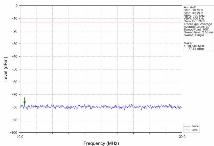
Band66 20MHz 16QAM HCH 1770MHz RB 1 0 NTV
