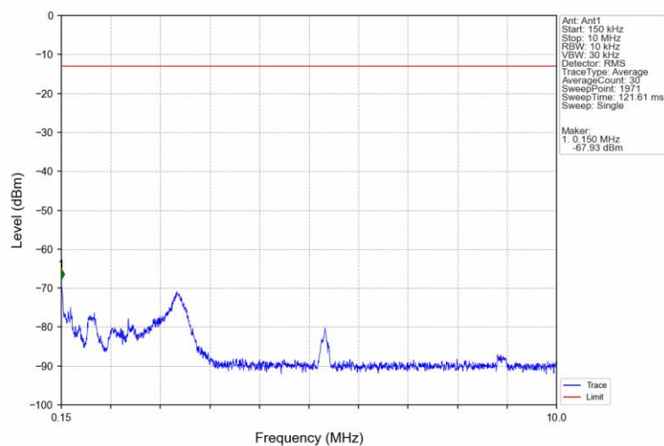
Band66 20MHz 16QAM LCH 1720MHz RB 1 0 NTV
