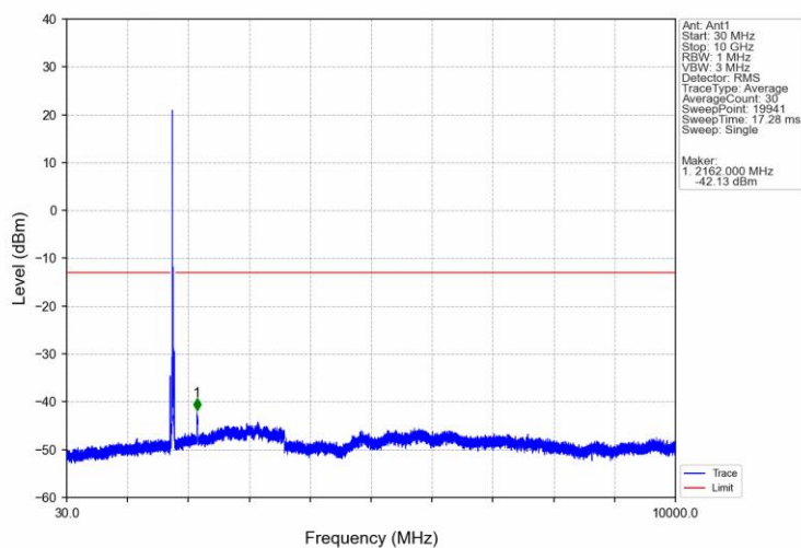
Band66 20MHz QPSK HCH 1770MHz RB 1 0 NTNV
