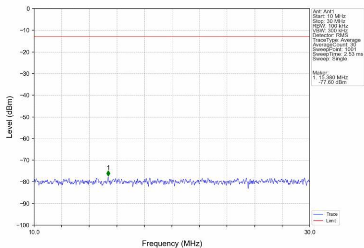
Band66 20MHz QPSK LCH 1720MHz RB 1 0 NTNV
