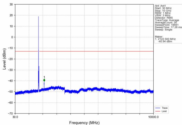
Band66 20MHz 16QAM LCH 1720MHz RB 1 0 NTV
