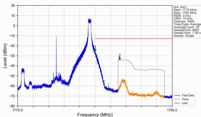
Band66 5MHz QPSK HCH 1777.5MHz RB 1 24 NTV
