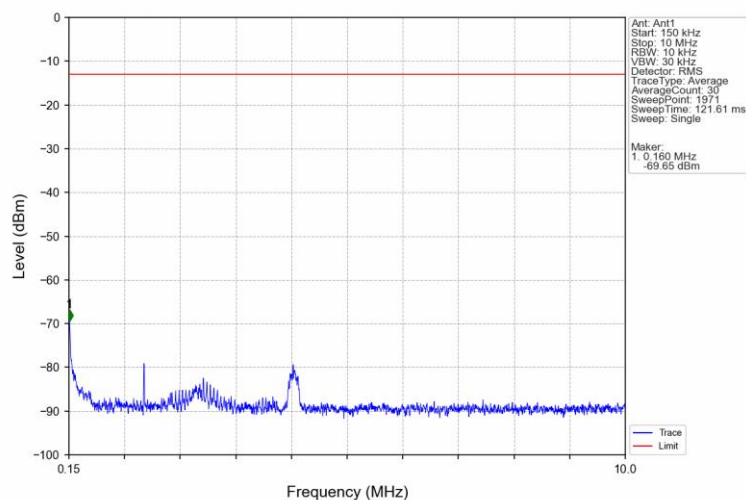
Band66 1.4MHz QPSK LCH 1710.7MHz RB 1 0 NTV
