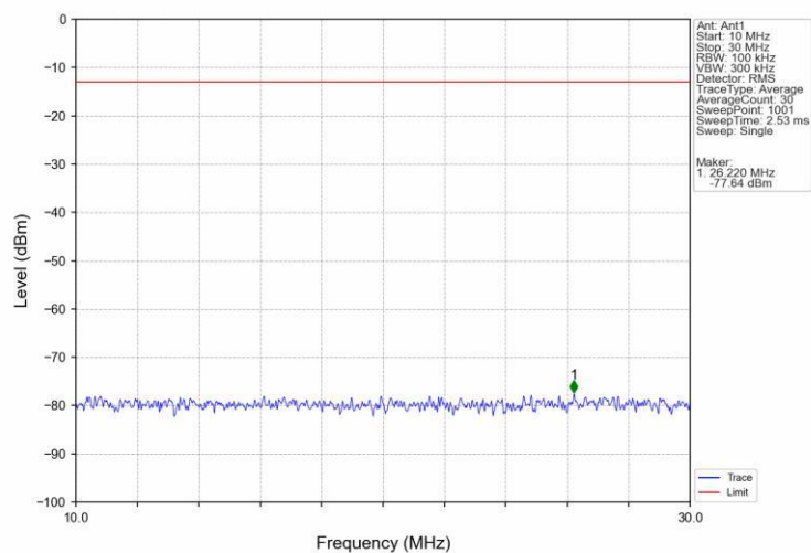
Band66 1.4MHz QPSK LCH 1710.7MHz RB 1 0 NTV
