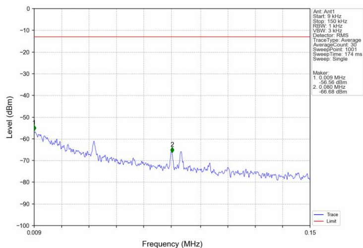
Band71 10MHz 16QAM MCH 680.5MHz RB 1 0 NTNV
