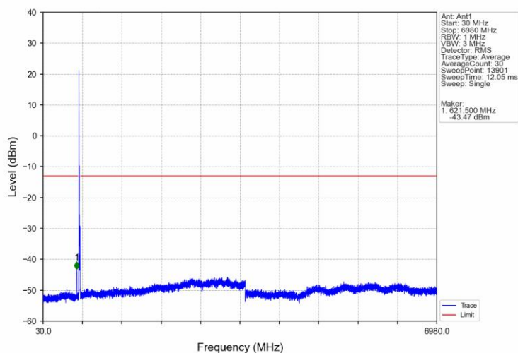
Band71 10MHz QPSK LCH 668MHz RB 50 0 NTN
