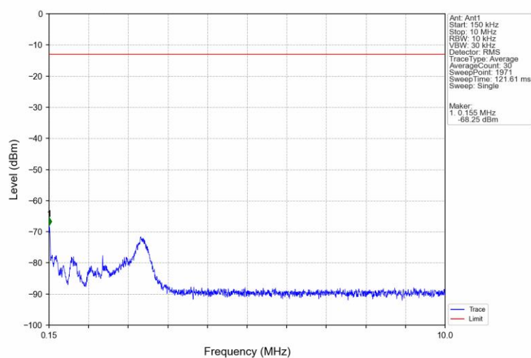
Band71 5MHz 16QAM MCH 680.5MHz RB 1 0 NTV
