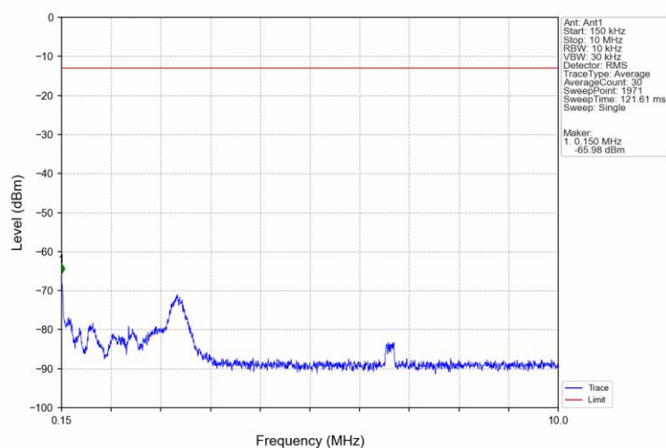
Band71_15MHz_QPSK_LCH_670.5MHz_RB_1_0_NTNV
