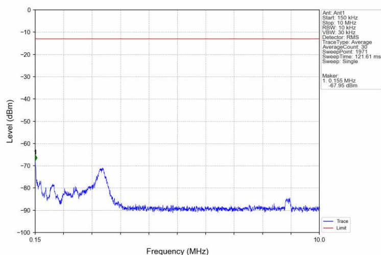
Band71 20MHz QPSK MCH 683MHz RB 1 0 NTNV
