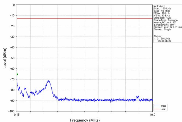
Band71 20MHz QPSK HCH 688MHz RB 1 0 NTNV
