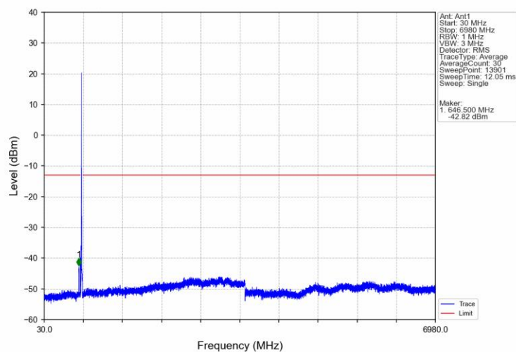
Band71 10MHz 16QAM HCH 693MHz RB 1 0 NTNV
