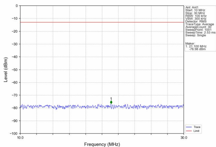
Band71_20MHz_QPSK_LCH_673MHz_RB_1_0 NTN
