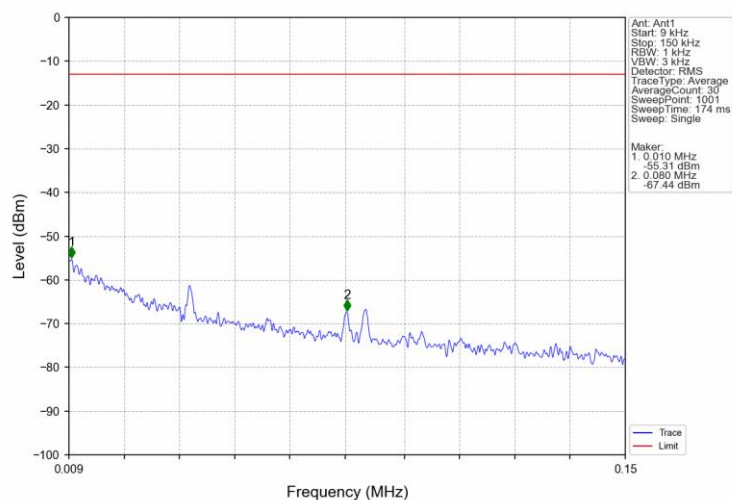
Band71 10MHz QPSK MCH 680.5MHz RB 1 0 NTV
