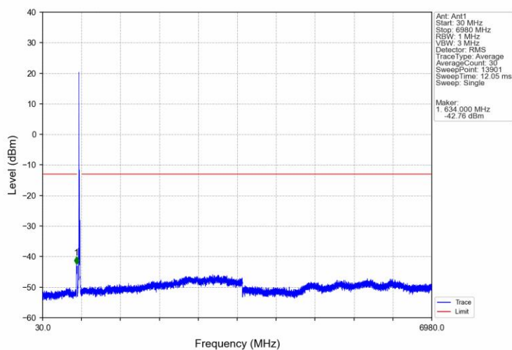
Band71 20MHz QPSK HCH 688MHz RB 1 0 NTNV
