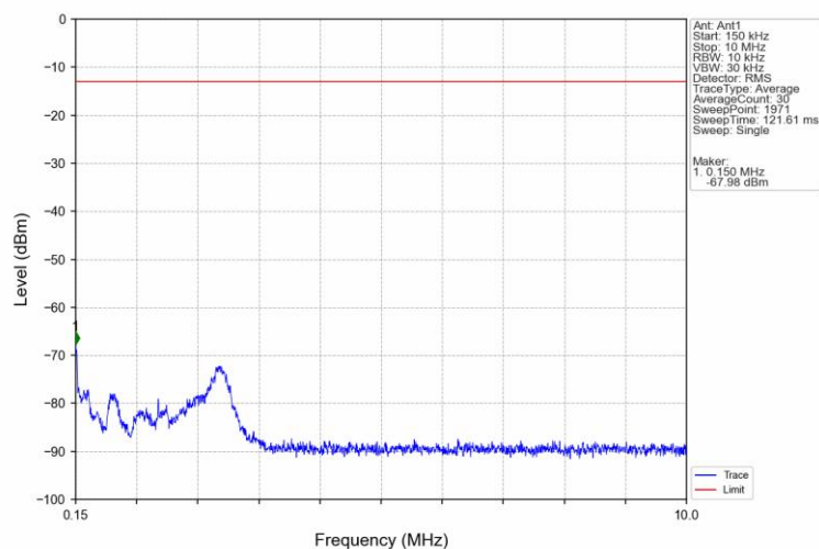
Band71 5MHz 16QAM LCH 665.5MHz RB 1 0 NTV
