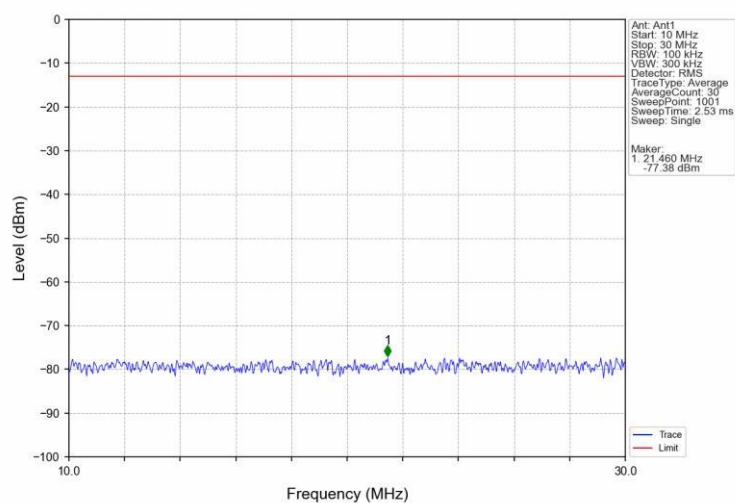
Band71_20MHz_16QAM_LCH_673MHz_RB_1_0_NTNV
