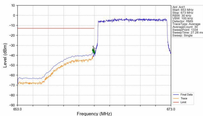
Band71 10MHz 16QAM LCH 668MHz RB 50 0 NTNV
