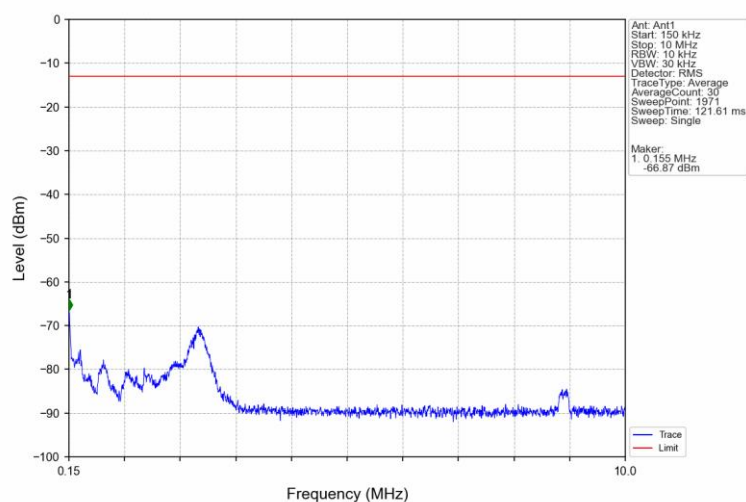
Band71_20MHz_16QAM_LCH_673MHz_RB_1_0_NTNV
