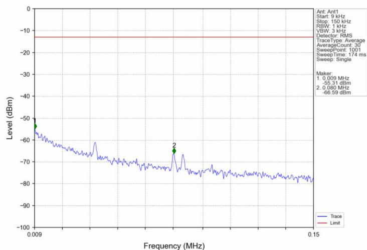
Band71 5MHz 16QAM HCH 695.5MHz RB 1 0 NTV
