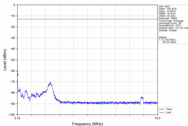
Band71_20MHz_QPSK_LCH_673MHz_RB_1_0 NTN
