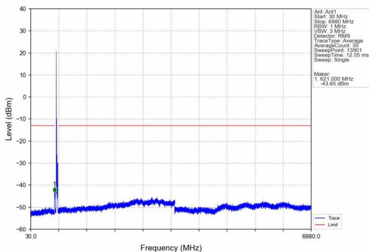
Band71_20MHz_QPSK_LCH_673MHz_RB_100_0_NTNV
