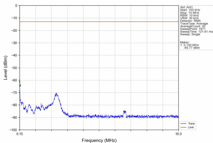
Band71 15MHz QPSK MCH 680.5MHz RB 1 0 NTV
