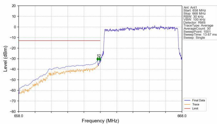
Band71 5MHz 16QAM LCH 665.5MHz RB 25 0 NTV
