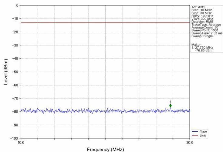
Band71 5MHz 16QAM MCH 680.5MHz RB 1 0 NTV
