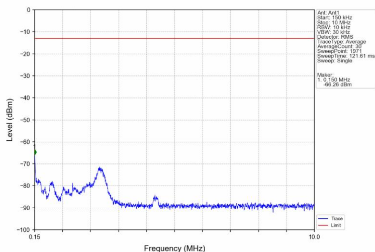
Band71 10MHz QPSK MCH 680.5MHz RB 1 0 NTV
