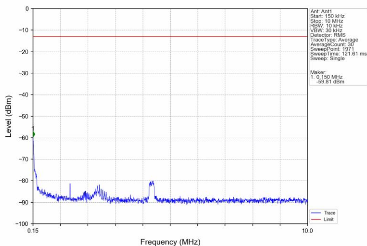
Band26a_10MHz_QPSK_LCH_819MHz_RB_1_0_NTNV
