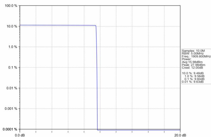
PCS1900 GSM HCH 1909.8MHz GSM NTN
