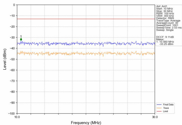
PCS1900 GSM HCH 1909.8MHz GSM NTN
