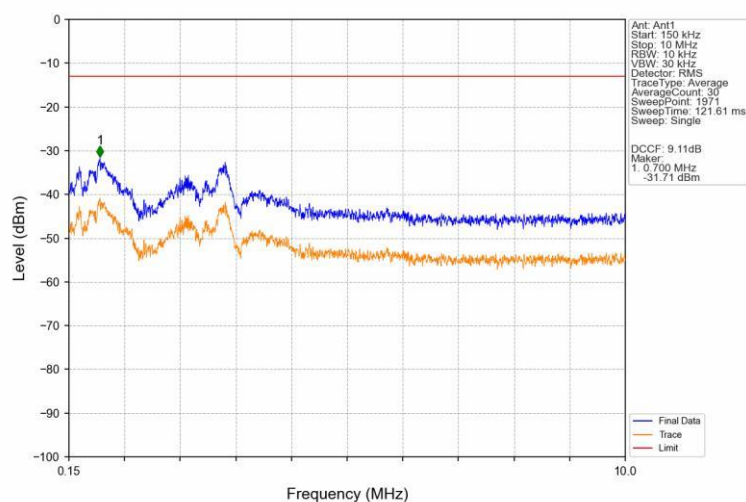
PCS1900 GSM HCH 1909.8MHz GSM NTN
