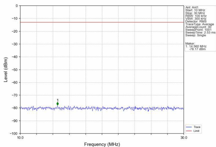
Band25 15MHz QPSK LCH 1857.5MHz RB 1 0 NTV
