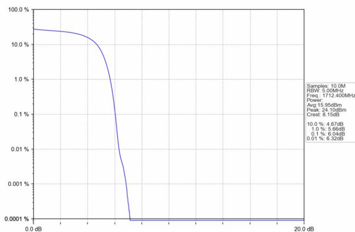
Band4 HSUPA LCH 1712.4MHz Subtest 1 NTVN
