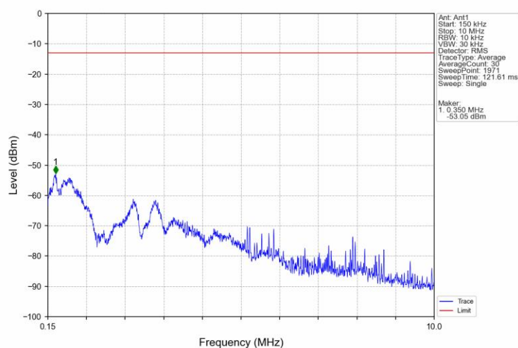
Band4_HSUPA_LCH_1712.4MHz_Subtest 1_NTNV
