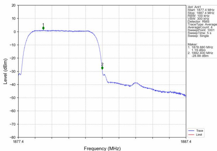
Band2_HSUPA_MCH_1880MHz_Subtest 1_NTNV
