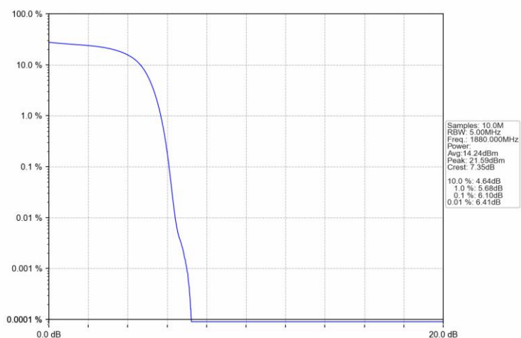
Band2_HSUPA_MCH_1880MHz_Subtest 1_NTNV
