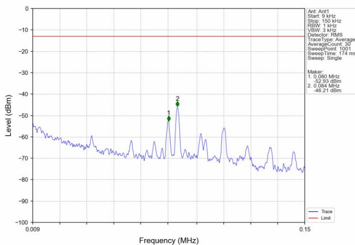
Band2_HSUPA_MCH_1880MHz_Subtest 1_NTNV
