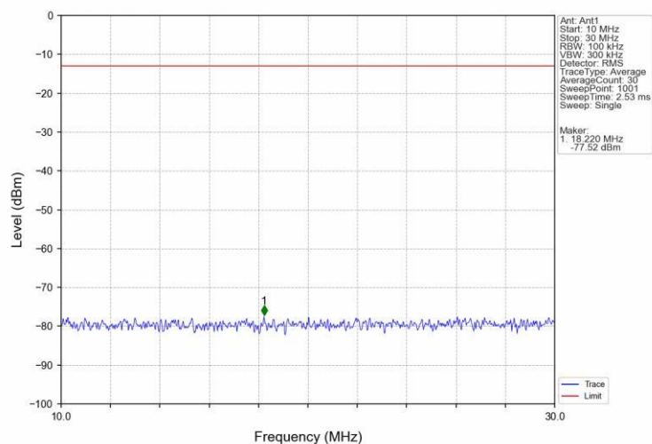
Band13 5MHz QPSK HCH 784.5MHz RB 1 0 NTN
