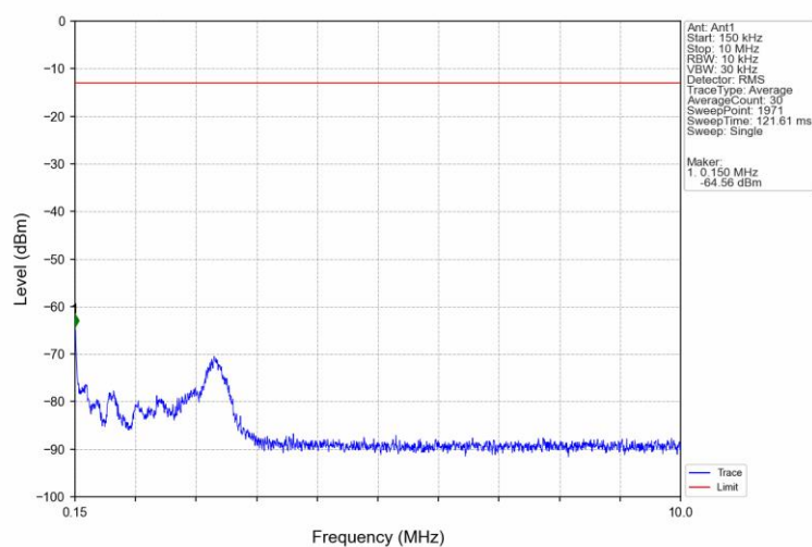
Band13 5MHz QPSK HCH 784.5MHz RB 1 0 NTN
