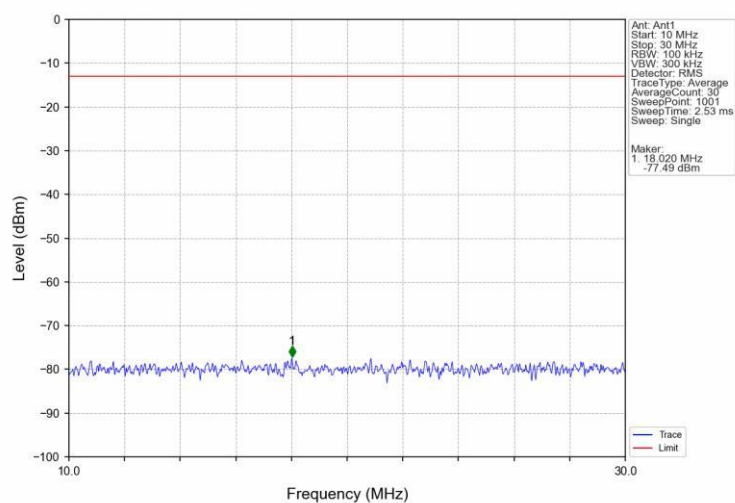
Band13 5MHz 16QAM LCH 779.5MHz RB 1 0 NTV
