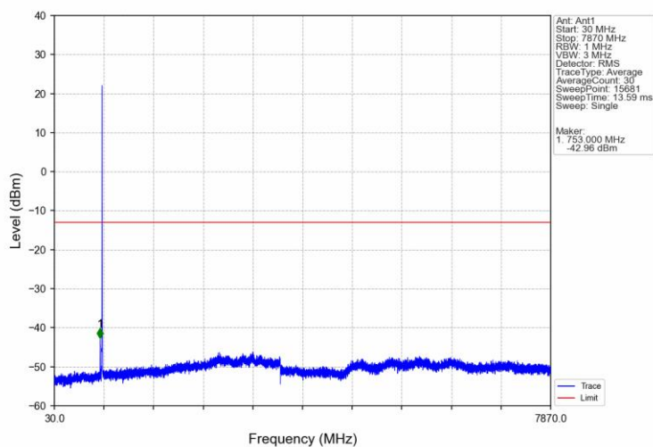
Band13 5MHz QPSK HCH 784.5MHz RB 1 0 NTN
