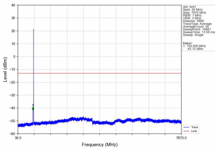
Band13 5MHz QPSK LCH 779.5MHz RB 25 0 NTNV
