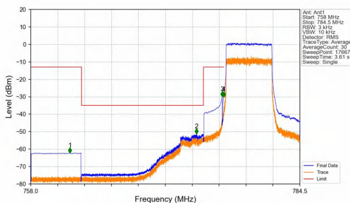
Band13 5MHz QPSK LCH 779.5MHz RB 25 0 NTNV
