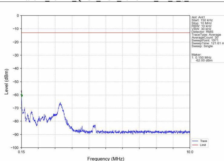
Band12 10MHz QPSK MCH 707.5MHz RB 1 0 NTV
