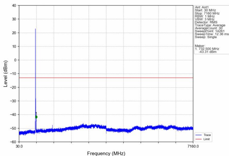
Band12 5MHz QPSK LCH 701.5MHz RB 25 0 NTNV
