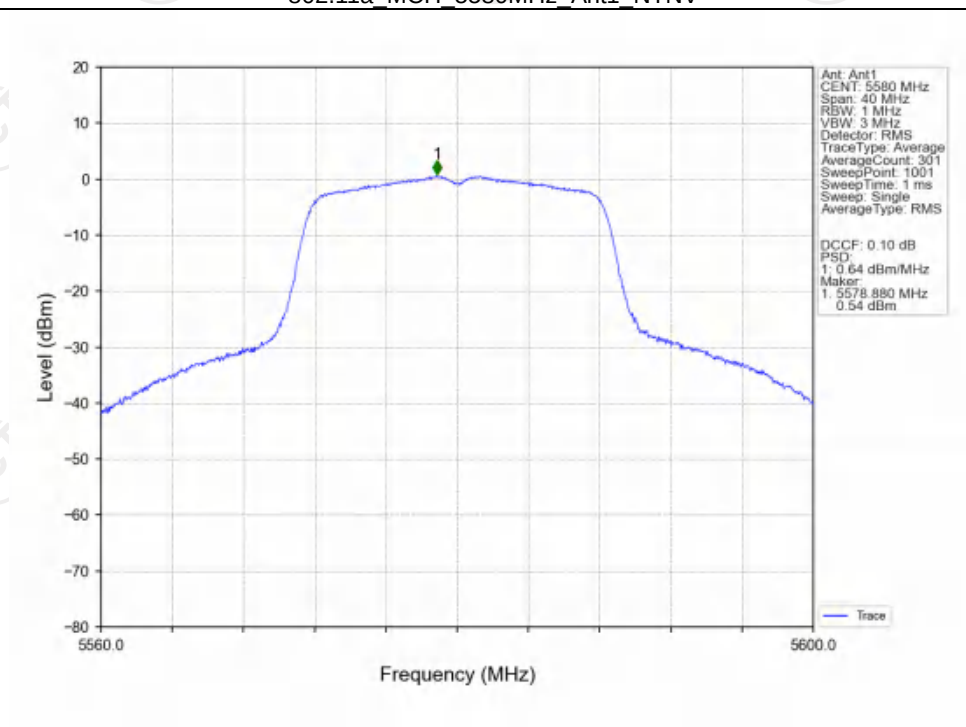
802.11a_MCH_5580MHz_Ant1_NTNV
