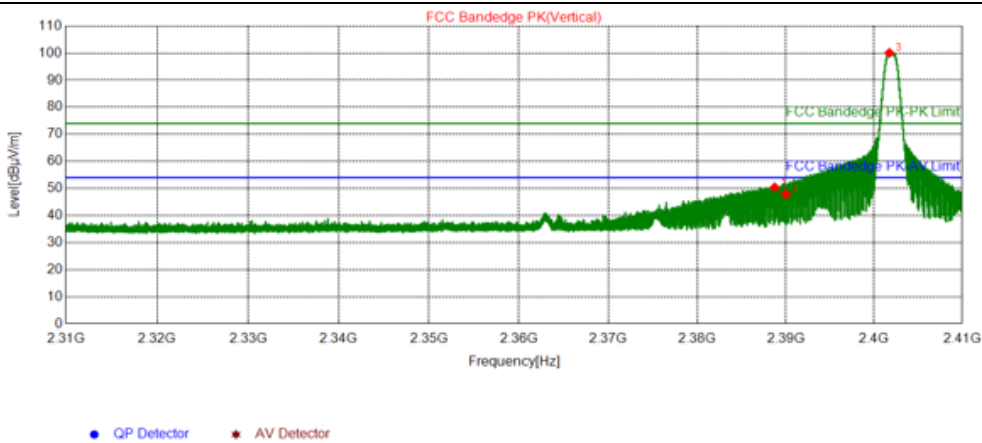
BLE_2402_Ant1/ Vertical
