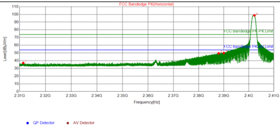
BLE_2402_Ant1/ Horizontal
