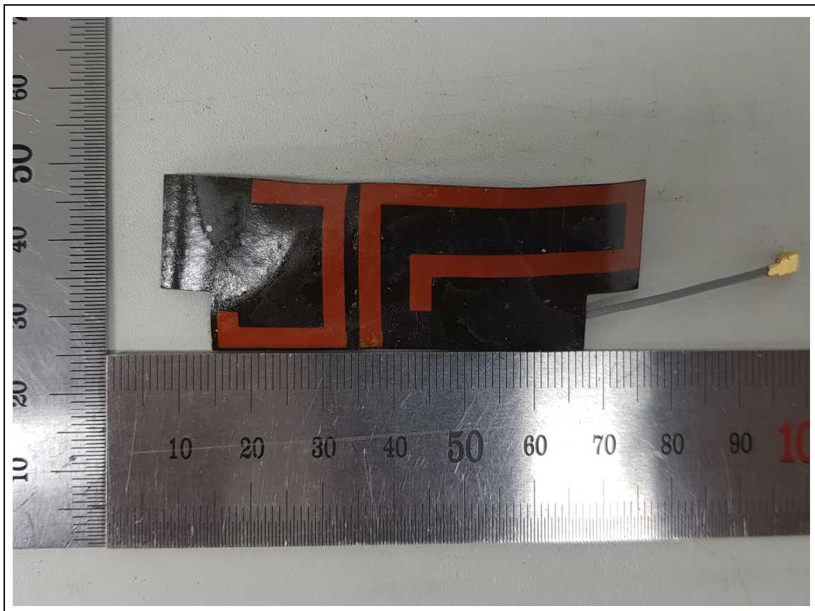
<WCDMA Antenna>
