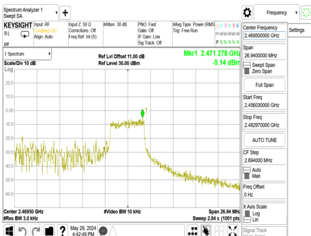
802.11ax_20MHz_Chain0_2462MHz_RU52_40
