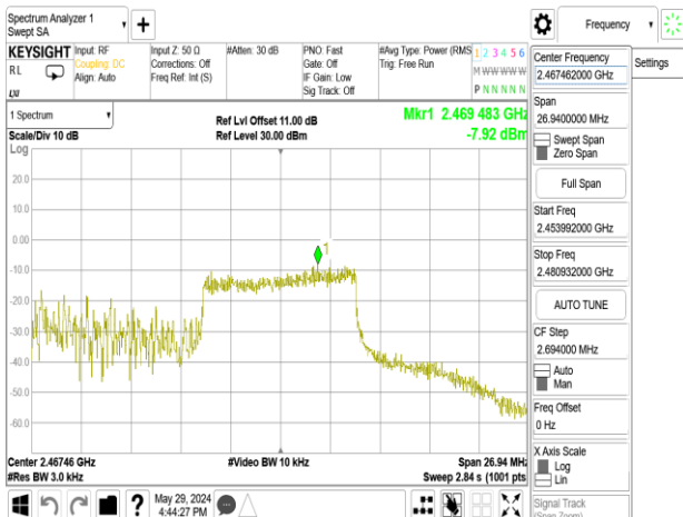
802.11ax_20MHz_Chain0_2462MHz_RU26_8
