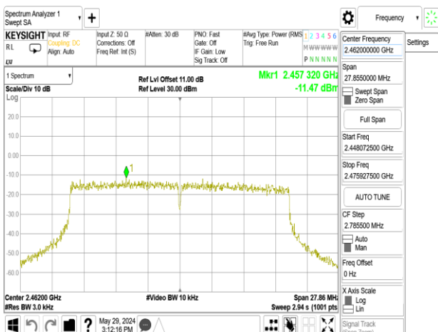
802.11ax_20MHz_Chain1_2462MHz
