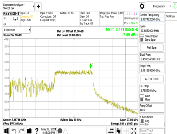
802.11ax_20MHz_Chain1_2462MHz_RU26_8
