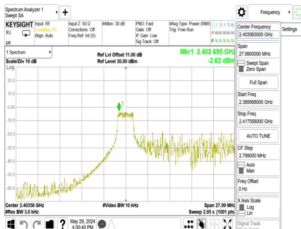
802.11ax_20MHz_Chain1_2412MHz_RU26_0
