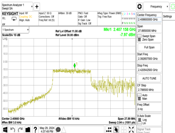
802.11ax_20MHz_Chain0_2412MHz_RU26_0
