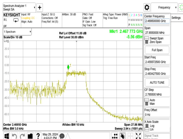
802.11ax_20MHz_Chain1_2462MHz_RU52_40
