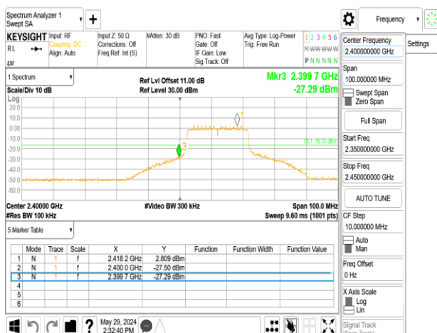
802.11ax_20MHz_Chain1_2412MHz
