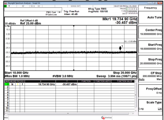
Band2_3MHz_QPSK_RB1_0_CH19185
