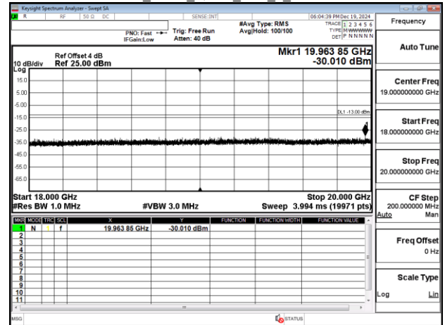
Band2_3MHz_QPSK_RB1_0_CH18900
