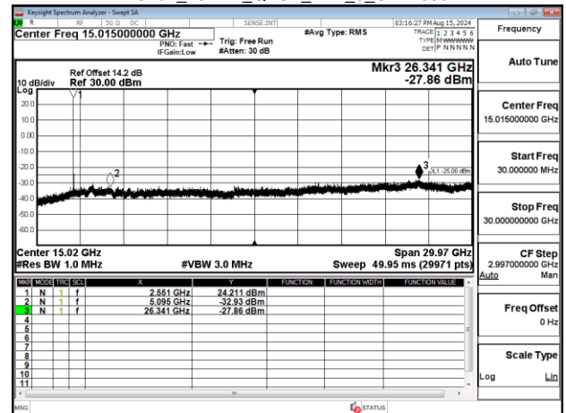
Band7_20MHz_QPSK_RB1_0_CH21350
