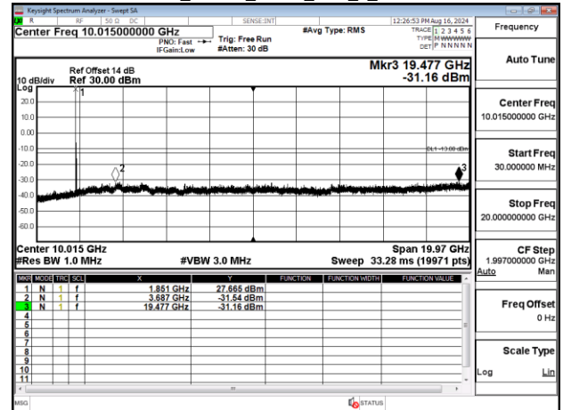
Band25_20MHz_QPSK_RB1_0_CH26140
