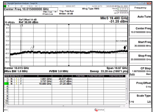
Band2_10MHz_QPSK_RB1_0_CH18900
