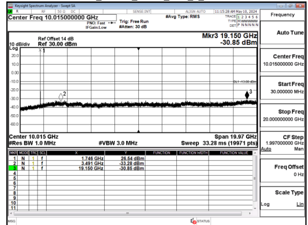
Band4_10MHz_QPSK_RB1_0_CH20350
