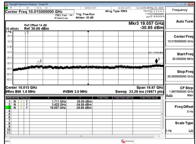
Band4_10MHz_QPSK_RB1_0_CH20175
