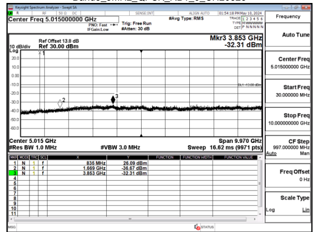
Band5_3MHz_QPSK_RB1_0_CH20635
