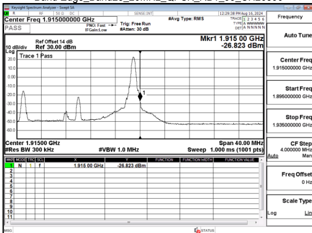
Band Edge_Band25_20MHz_QPSK_RB1_99_CH26590
