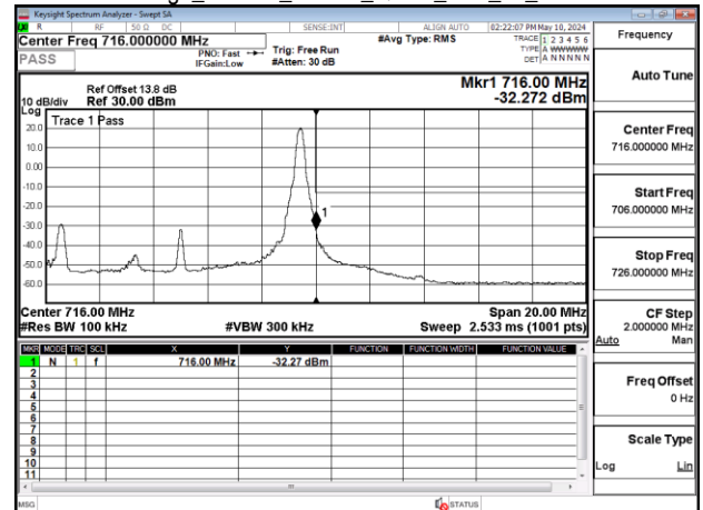
Band Edge_Band12_10MHz_QPSK_RB1_49_CH23130
