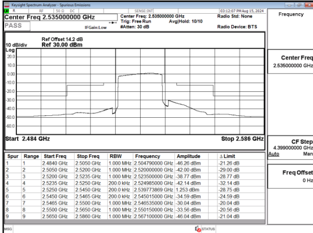
Emission Mask Band7_20MHz_QPSK_RB100_0_CH21100
