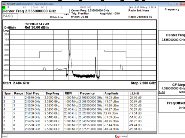
Emission Mask_Band7_20MHz_QPSK_RB1_0_CH21100
