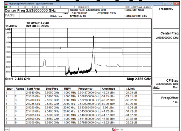
Emission Mask_Band7_20MHz_QPSK_RB1_99_CH21100
