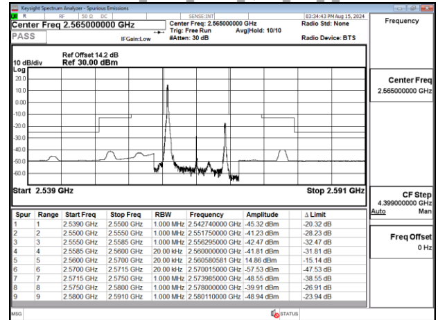
Emission Mask_Band7_10MHz_QPSK_RB1_49_CH20800
