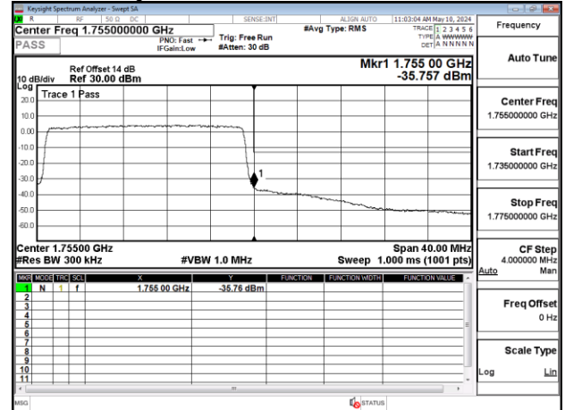
Band Edge_Band4_20MHz_QPSK_RB100_0_CH20300
