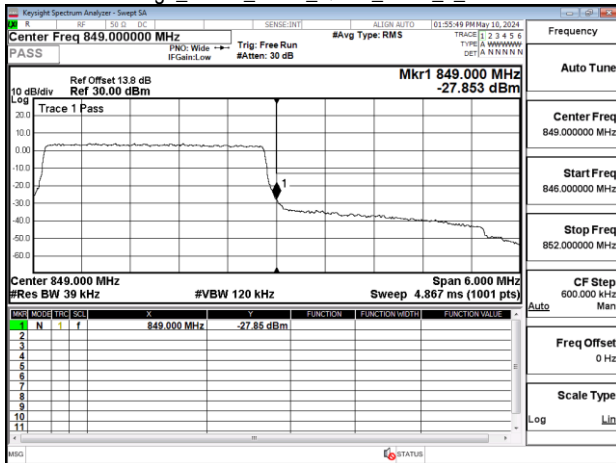
Band Edge_Band5_5MHz_QPSK_RB1_0_CH20425
