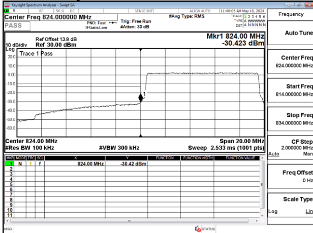
Band Edge_Band5_10MHz_QPSK_RB50_0_CH20450
