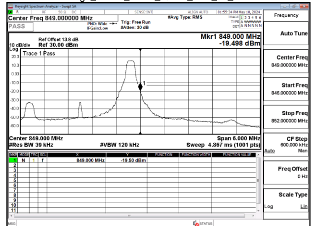
Band Edge_Band5_3MHz_QPSK_RB1_14_CH20635
