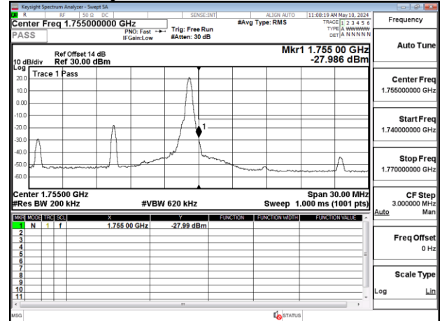
Band Edge_Band4_15MHz_QPSK_RB1_74_CH20325
