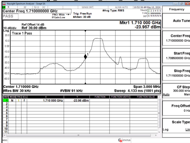
Band Edge_Band4_1.4MHz_QPSK_RB1_5_CH20393
