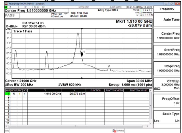
Band Edge_Band2_15MHz_QPSK_RB1_74_CH19125
