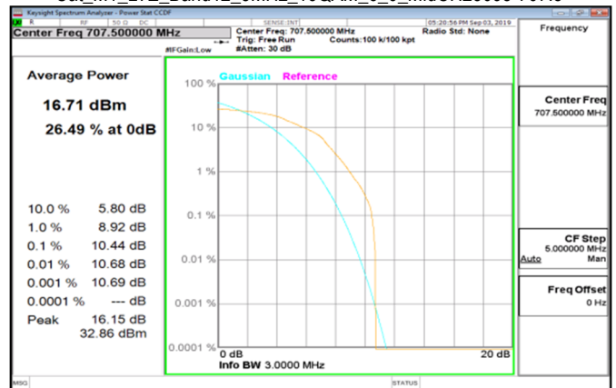
Cat M1 LTE_Band12_3MHz_16QAM_6_0_MidCH23095-707.5
