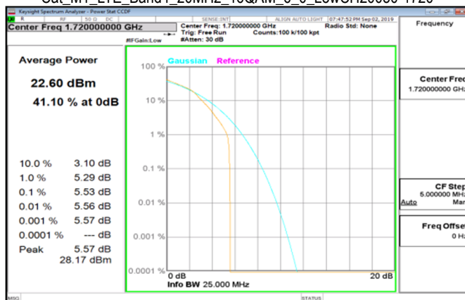
Cat_M1_LTE_Band4_20MHz_16QAM_6_0_LowCH20050-1720
