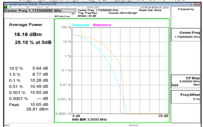
Cat M1 LTE_Band4_3MHz_16QAM_6_0_MidCH20175-1732.5
