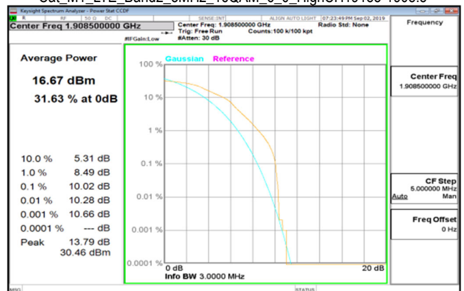
Cat M1 LTE_Band2_3MHz_16QAM_6_0_HighCH19185-1908.5
