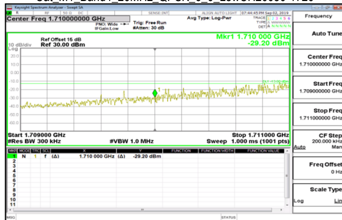
Cat_M1_Band4_20MHz_QPSK_6_0_LowCH20050-1720
