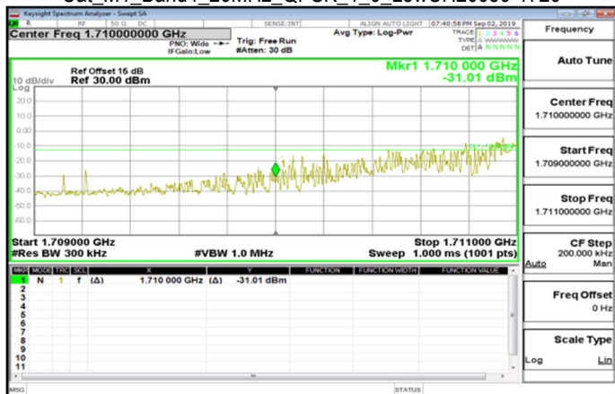
Cat_M1_Band4_20MHz_QPSK_1_0_LowCH20050-1720
