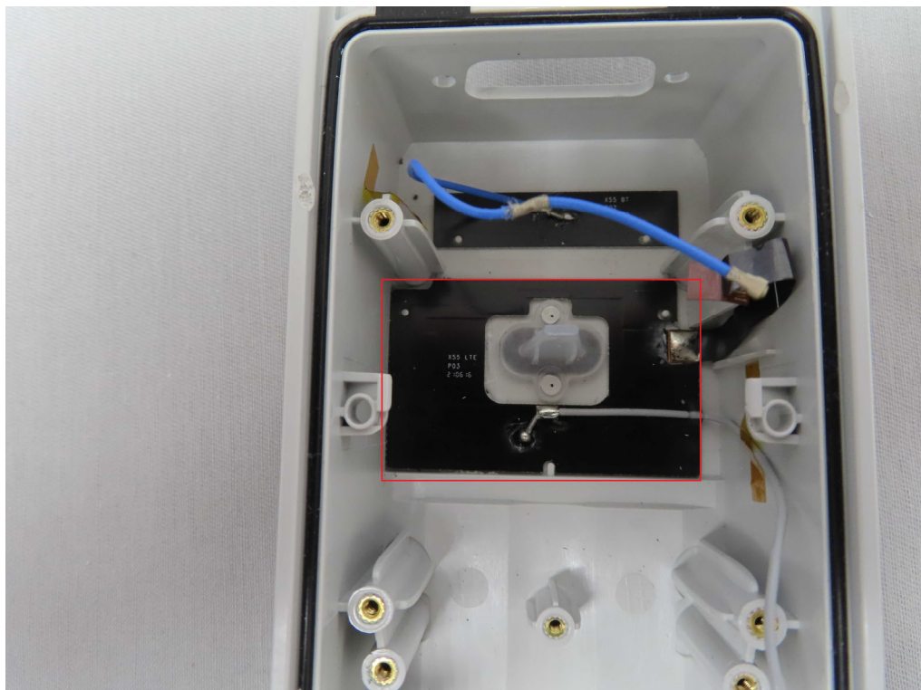
WWAN Antenna
