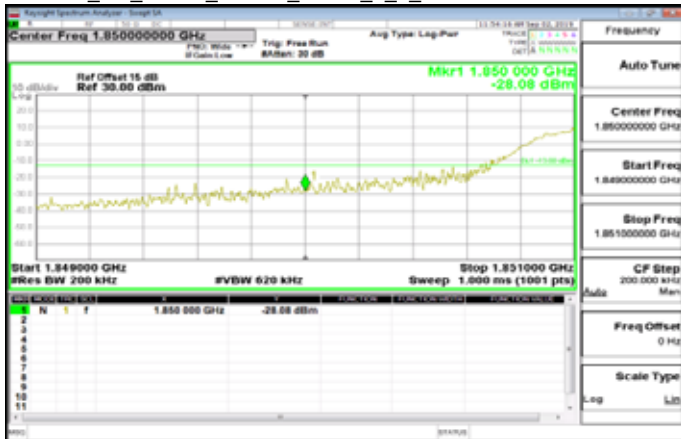
Cat_M1_Band2_15MHz_QPSK_6_0_LowCH18675-1857.5
