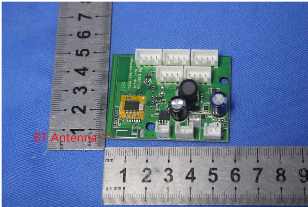
BLE Antenna
