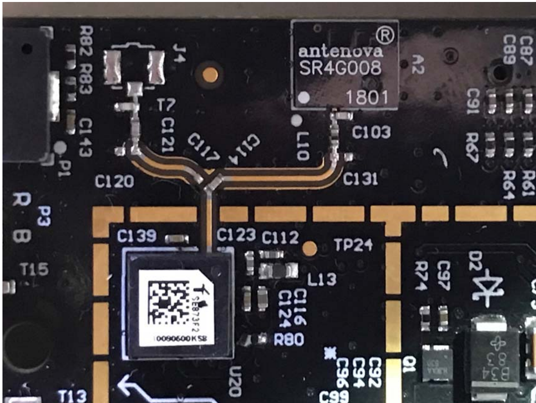
GNSS chip
