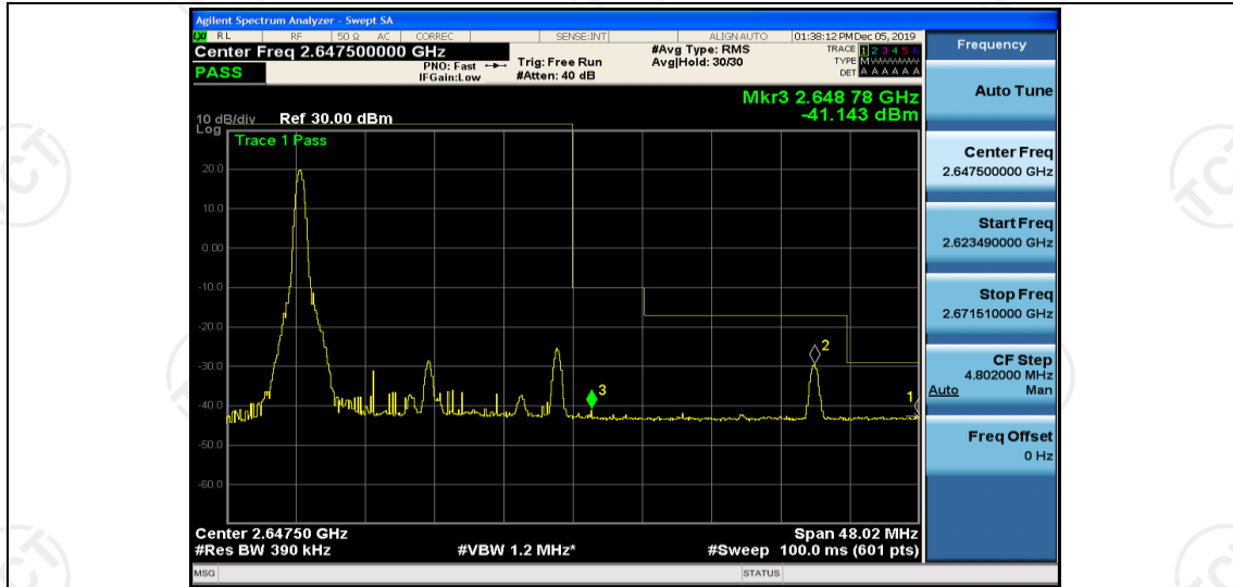
Band41-20MHz-QPSK-41065-100RB#0
