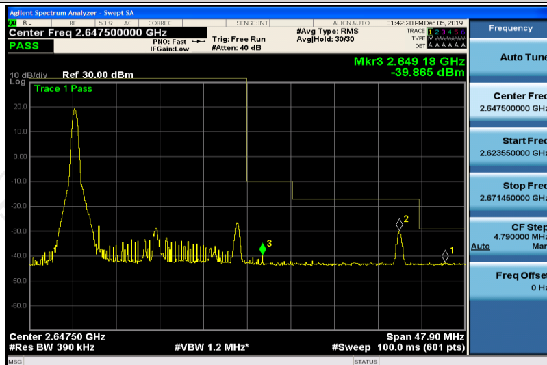
Band41-20MHz-16QAM-41065-1RB#99
