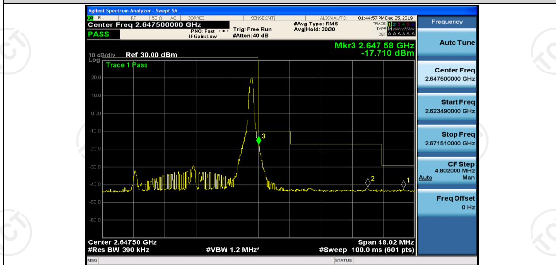
Band41-20MHz-QPSK-41065-1RB#0
