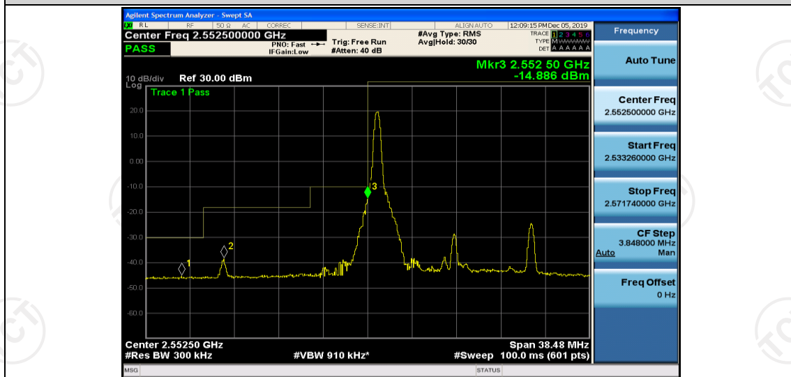
Band41-15MHz-16QAM-40290-1RB#74
