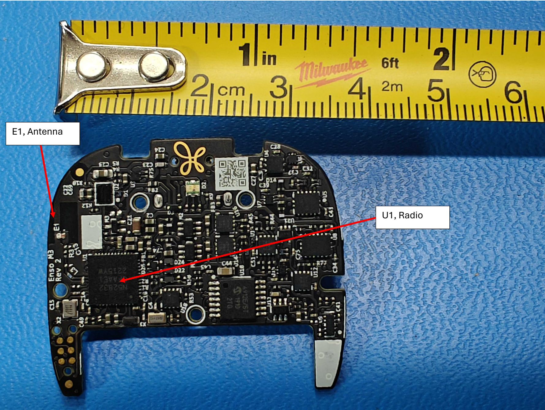
Enso 3 Device PCBA, Top
