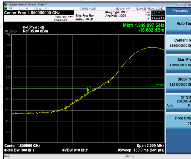
Band2-15MHz-16QAM-18675-1RB#74
